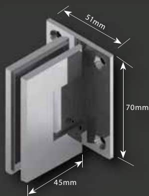
CMES1 - Wall Hung Hinge
