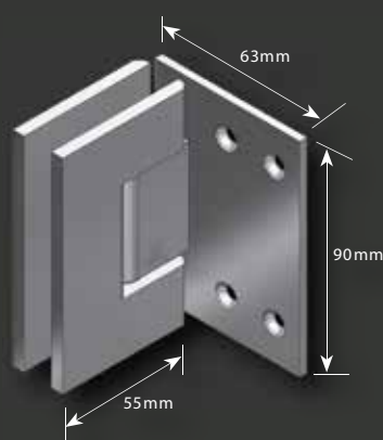
ES1-EXT - Wall Hung Hinge
