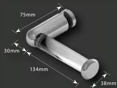
TRH1 - Toilet Roll Holder
